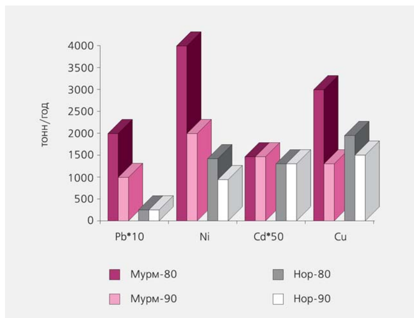
Эмиссия тяжелых металлов с территорий Мурманской обл. и района Норильска в 1980-х и 1990-х годах (значения для Pb и Cd увеличены в 10 и 50 раз соответственно).
